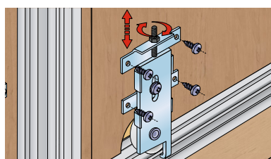
Montáž dolního vozíku Připevnit pevnou část. Připevnit pohyblivou část. Výškově seřídít.
