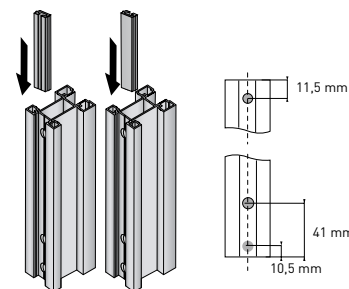
Vrtání úchytkového profilu
