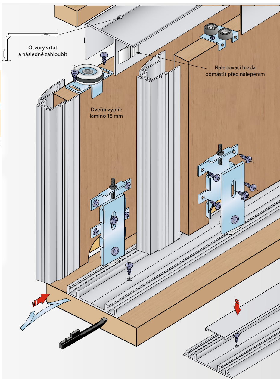
Montáž dolního vozíku Připevnit pevnou část. Připevnit pohyblivou část. Výškově seřídít.
