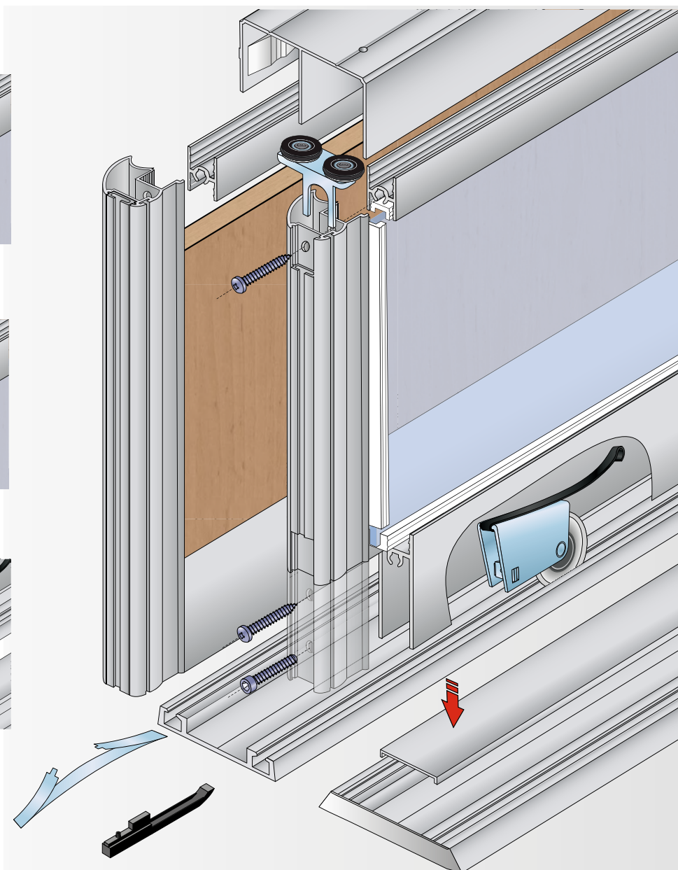
Montáž horního vozíku S55A Zasunout vozík do svislého profilu a zajistit šroubem.
