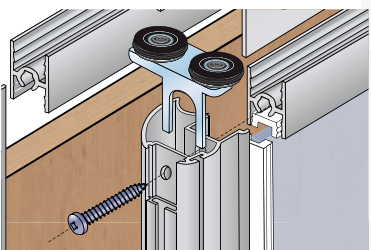
Montáž horního vozíku S55B Zasunout vozík do svislého profilu a zajistit šroubem.
