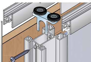
Montáž horního vozíku S55A Zasunout vozík do svislého profilu a zajistit šroubem.
