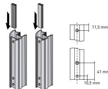
Montáž profilu S17
