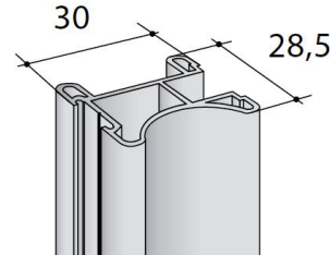
Madlo S22 - stříbrný elox
