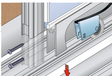
Montáž spodního vozíku Spodní vozík nasunout do spodního profilu a zajistit šroubem.
