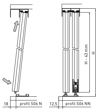
Sada S55B
