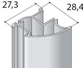
Madlo S17 - stříbrný elox
