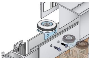
Montáž horního vozíku Nasadit vozík a našroubovat 2 vruty do podélných otvorů vozíku.
