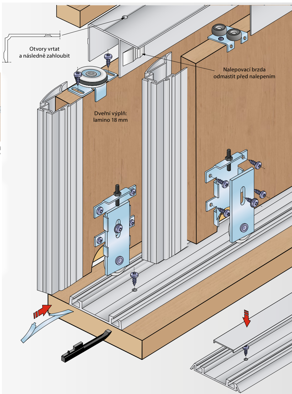
Montáž dolního vozíku Připevnit pevnou část. Připevnit pohyblivou část. Výškově seřídit.
