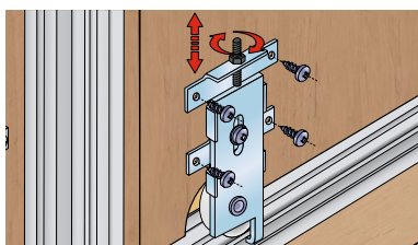
Montáž dolního vozíku Připevnit pevnou část. Připevnit pohyblivou část. Výškově seřídit.
