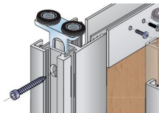
Montáž horního vozíku Zasunout vozík do svislého profilu a zajistit šroubem.
