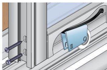
Montáž spodního vozíku Spodní vozík nasunout do spodního profilu a zajistit šroubem. Pomocí imbusového klíče výškově seřídit.
