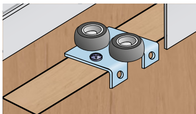
Montáž horního vozíku – dvojkolečko Nasadit vozík a našroubovat 2 vruty.
